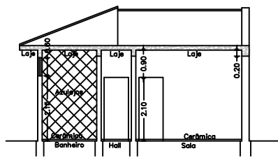
CORTE AA
