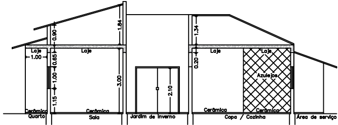
CORTE BB
