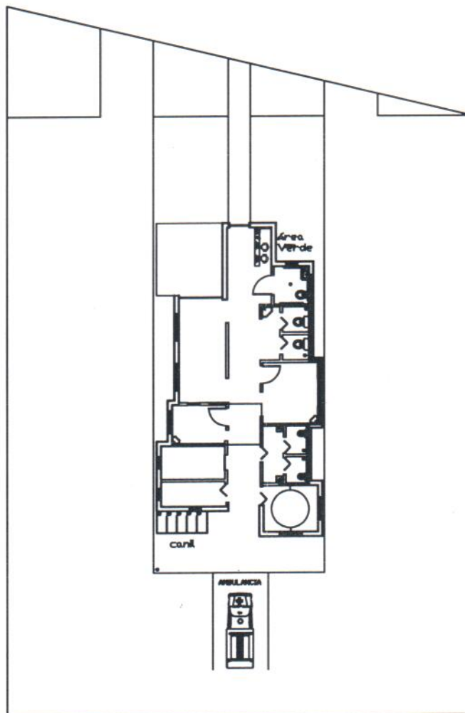
Planta Baixa Esc: 1:100
