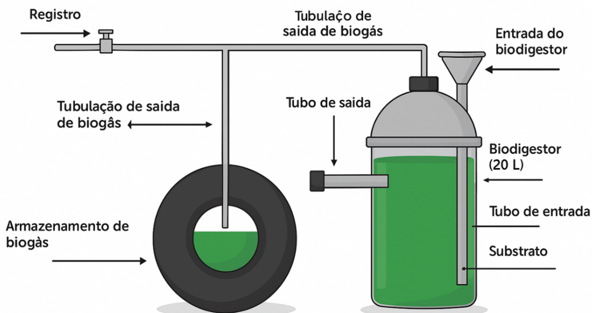
Figura 1. Esquema e estrutura física do biodigestor
