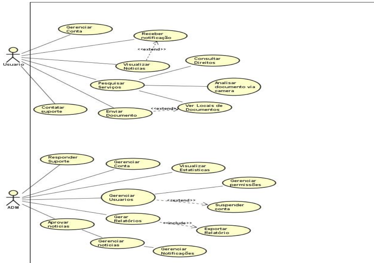
Figura 7: Caso de Uso
