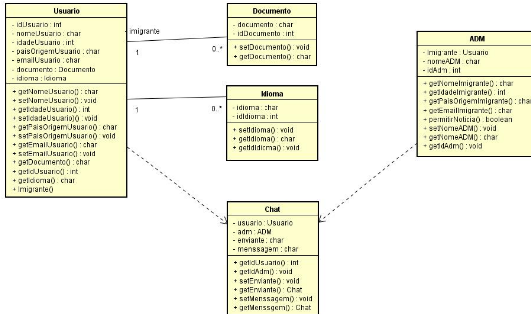
Figura 8: Classes e Objetos
