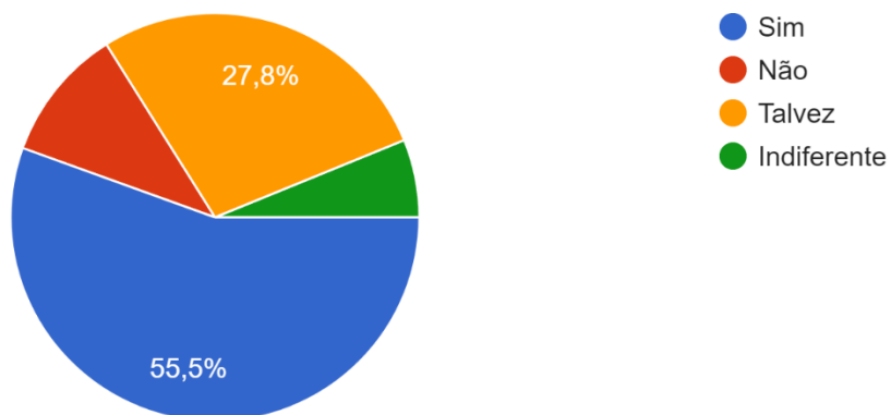
Figura 5: gráfico de levantamentos de dados: pergunta 5
