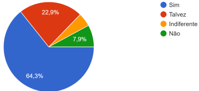
Figura 6: gráfico de levantamentos de dados: pergunta 6
