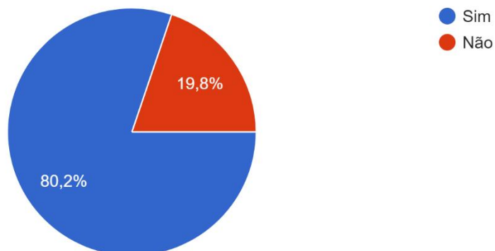
Figura 4: gráfico de levantamentos de dados: pergunta 4
