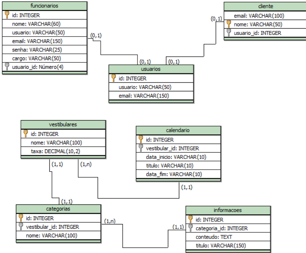
ANEXO B – Diagrama de entidade.
