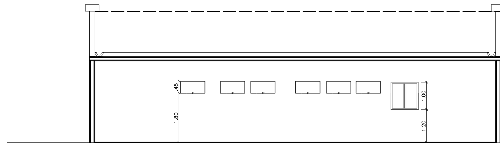
3 FACHADA LATERAL ESQUERDA CONVENIÊNCIA ESCALA 1:75
