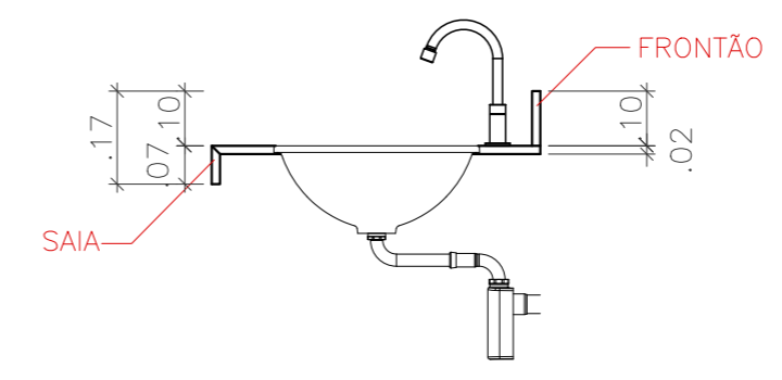
BANCADA W.C.1
