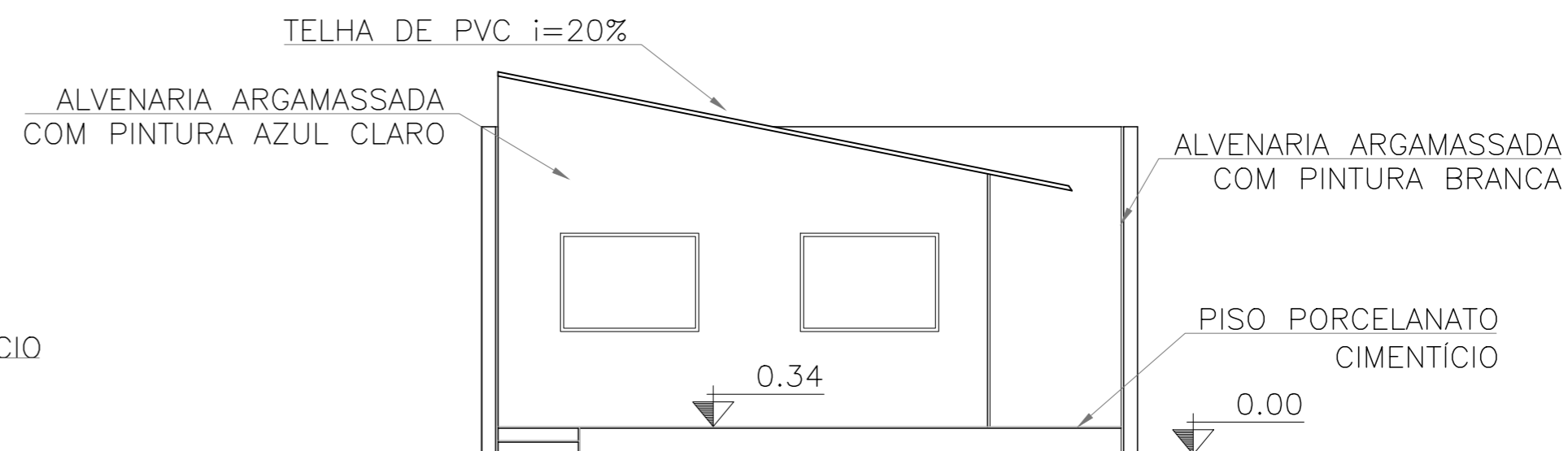
VISTA TRASEIRA ESCALA 1:75
