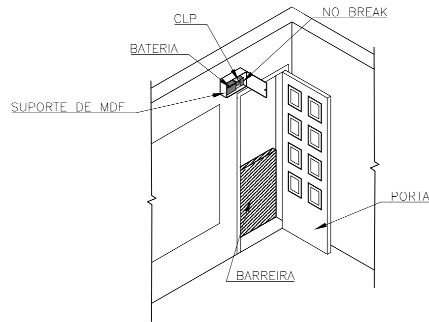
COMPORTA AUTOMÁTICA ISOMÉTRICA DIREITA ESCALA 1:20
