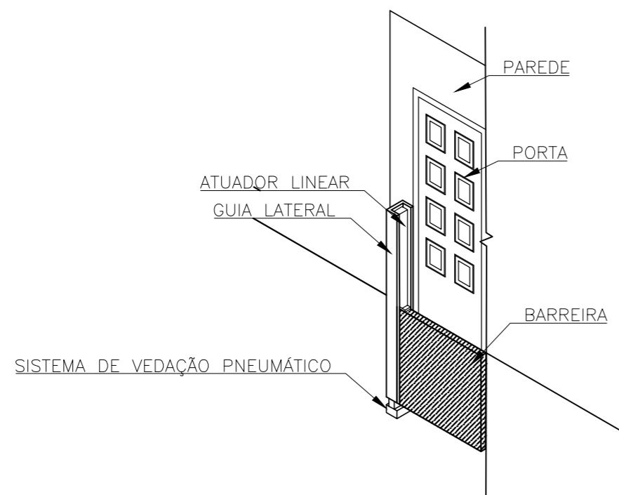
COMPORTA AUTOMÁTICA ISOMÉTRICA ESQUERDA ESCALA 1:20
