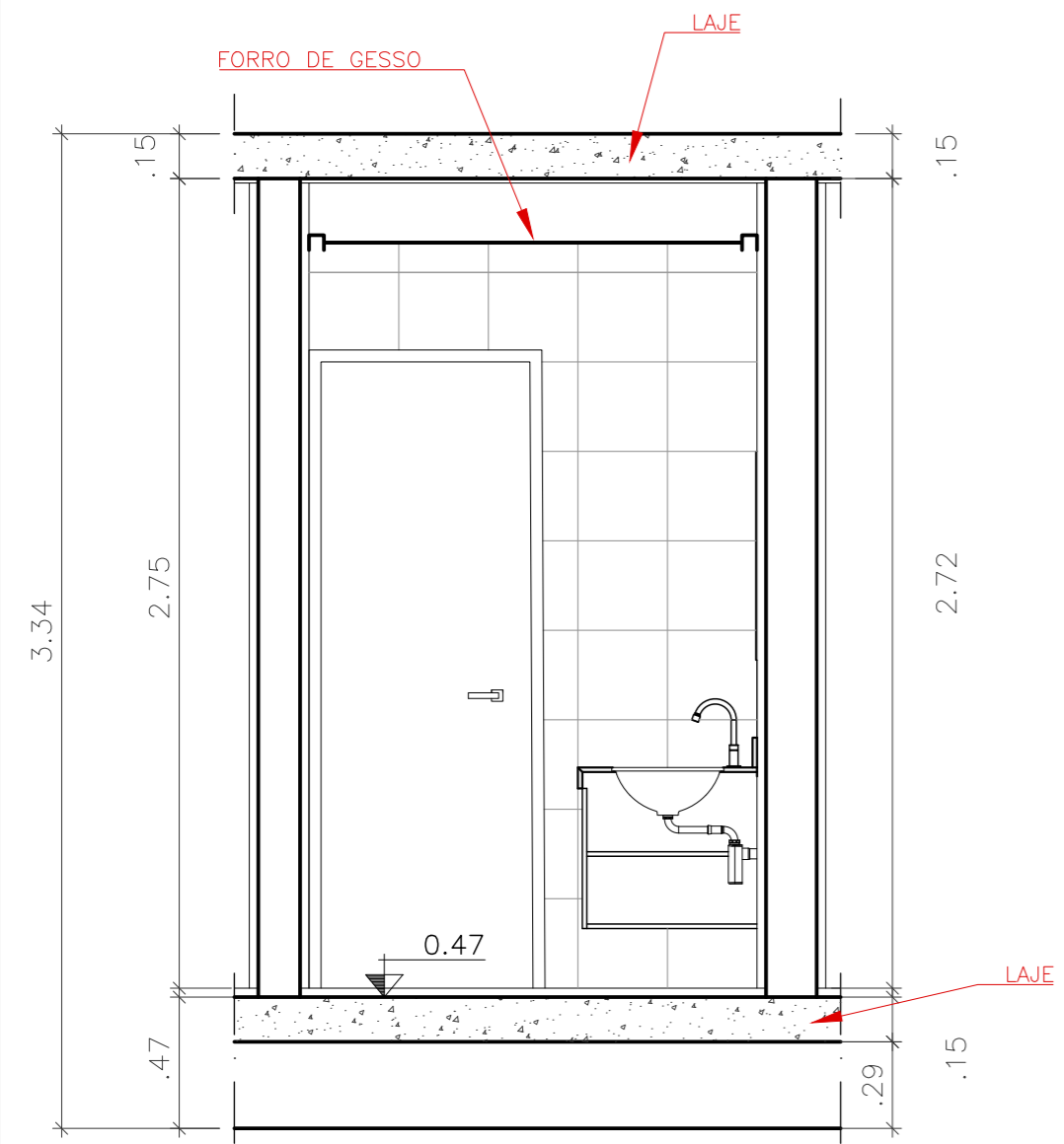
CORTE C:C
