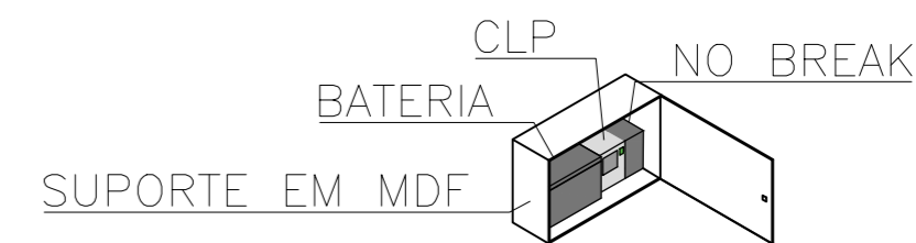
COMPORTA AUTOMÁTICA DET. SUPORTE ESCALA 1:20
