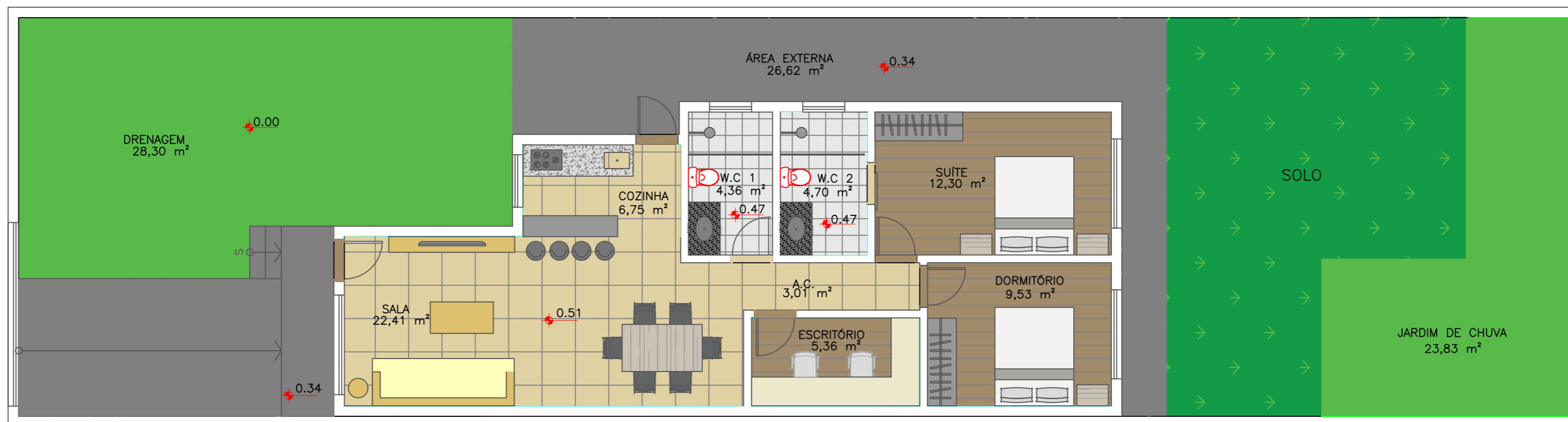
PLANTA HUMANIZADA
