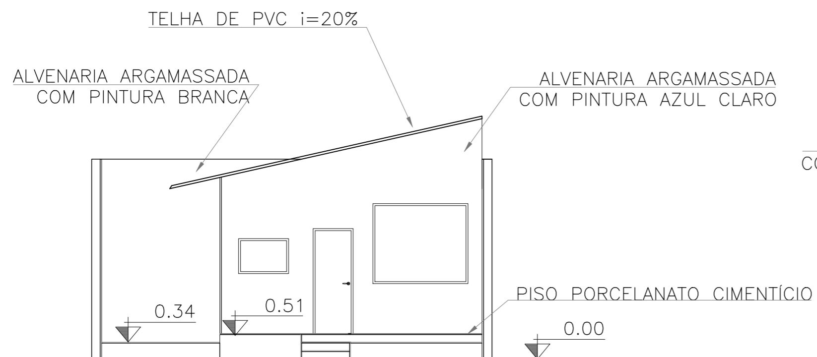
VISTA FRONTAL ESCALA 1:75
