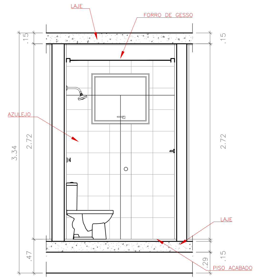
CORTE B:B
