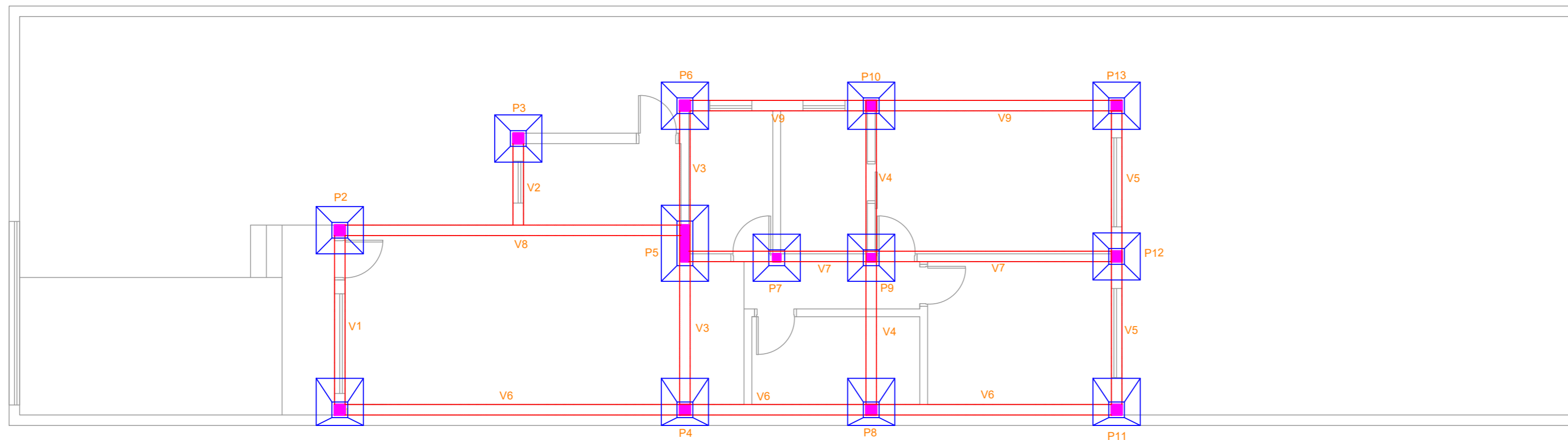
PLANTA ESTRUTURAL ESCALA 1:75
