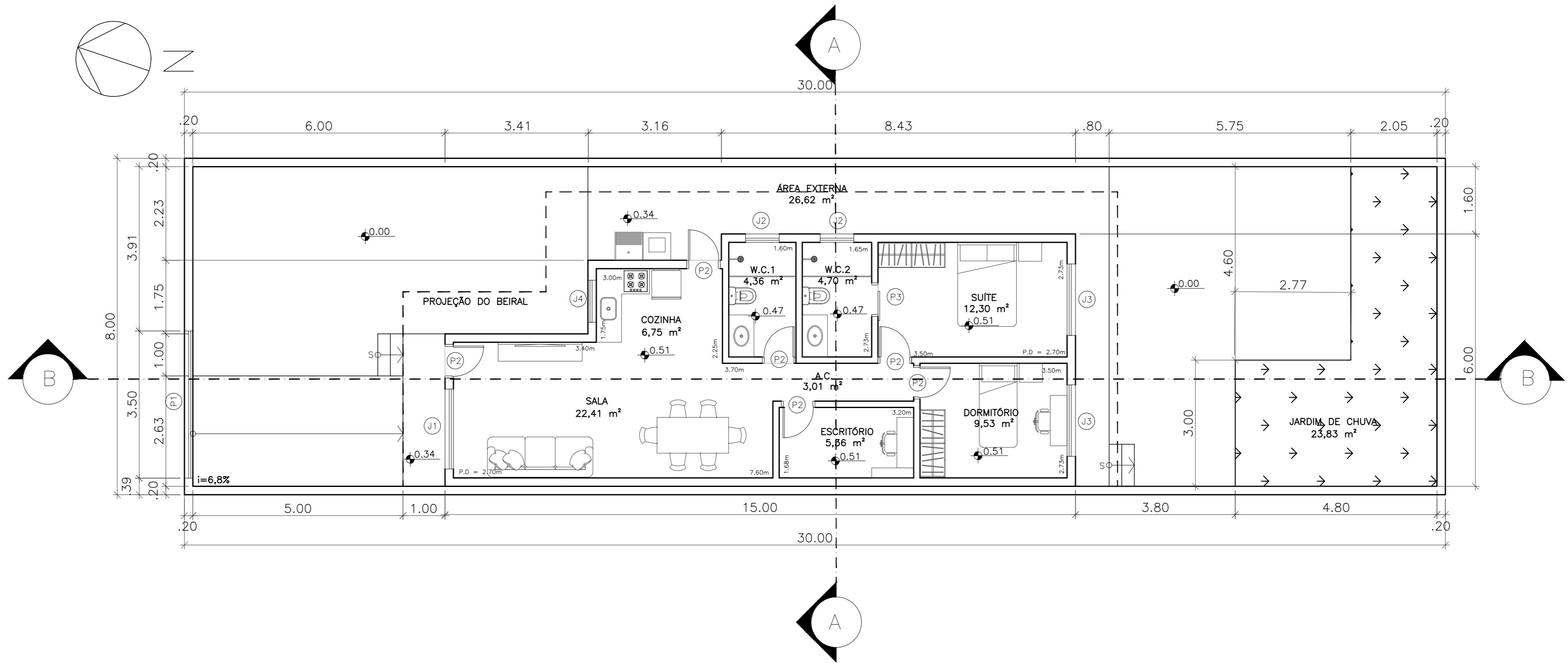
PLANTA BAIXA ESCALA 1:75
