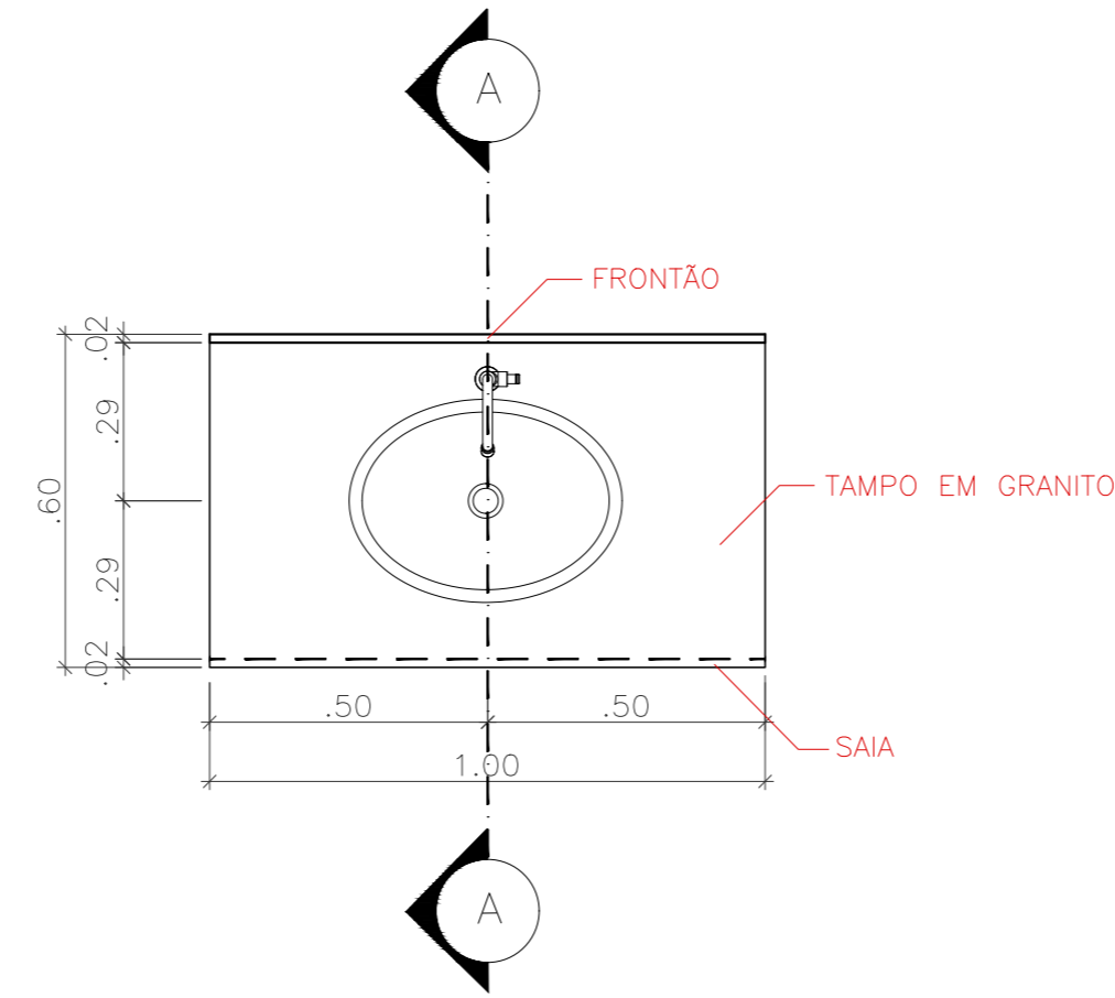
BANCADA W.C.1
