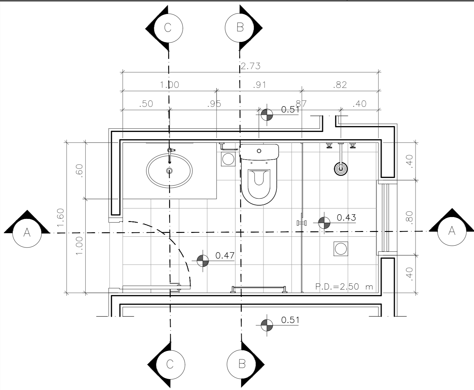
PLANTA DO W.C. 1
