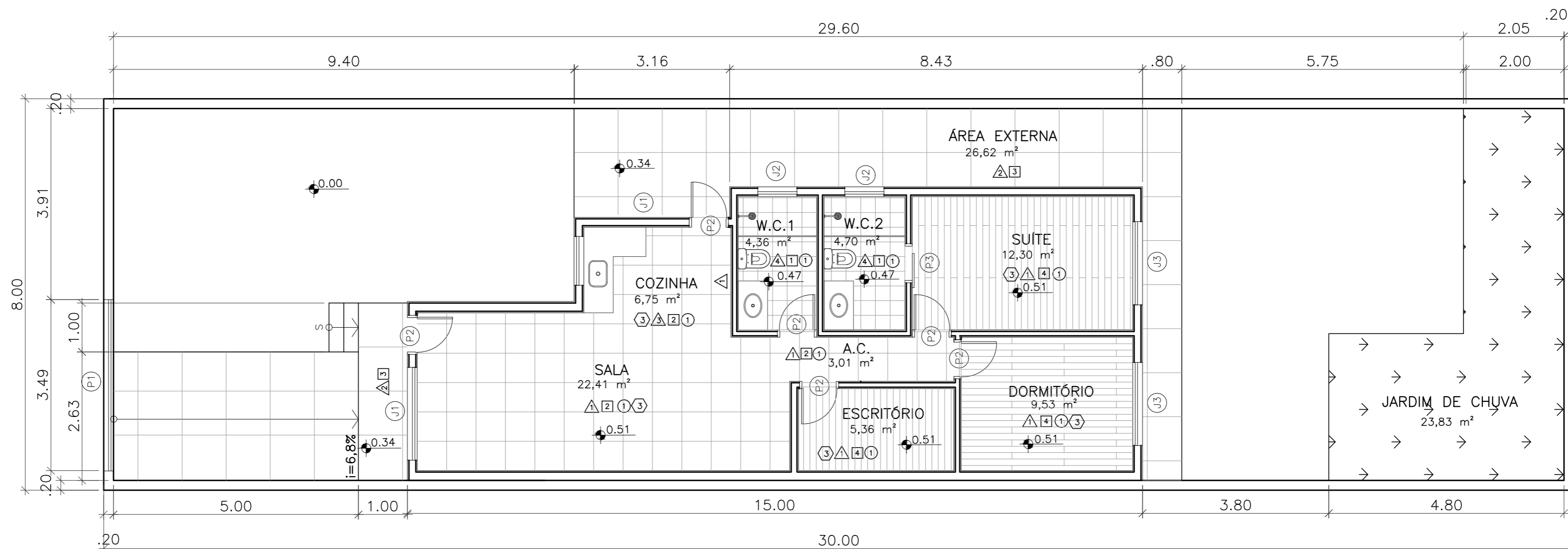
PLANTA BAIXA ESCALA 1:75
