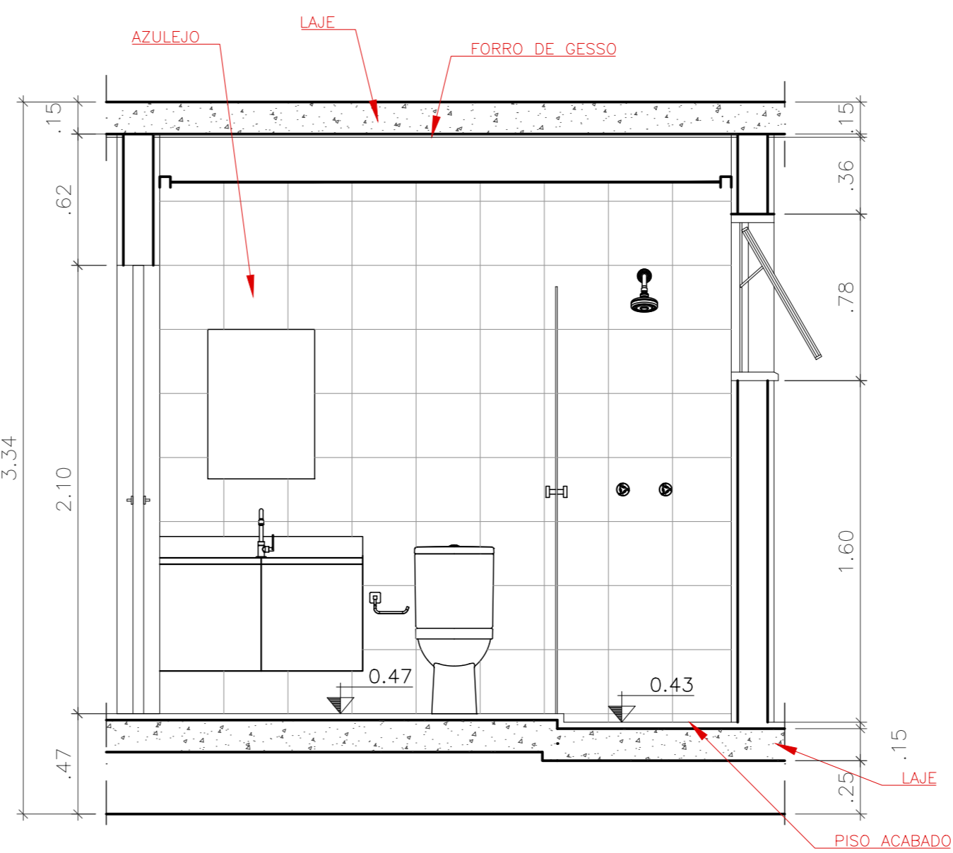
CORTE A:A
