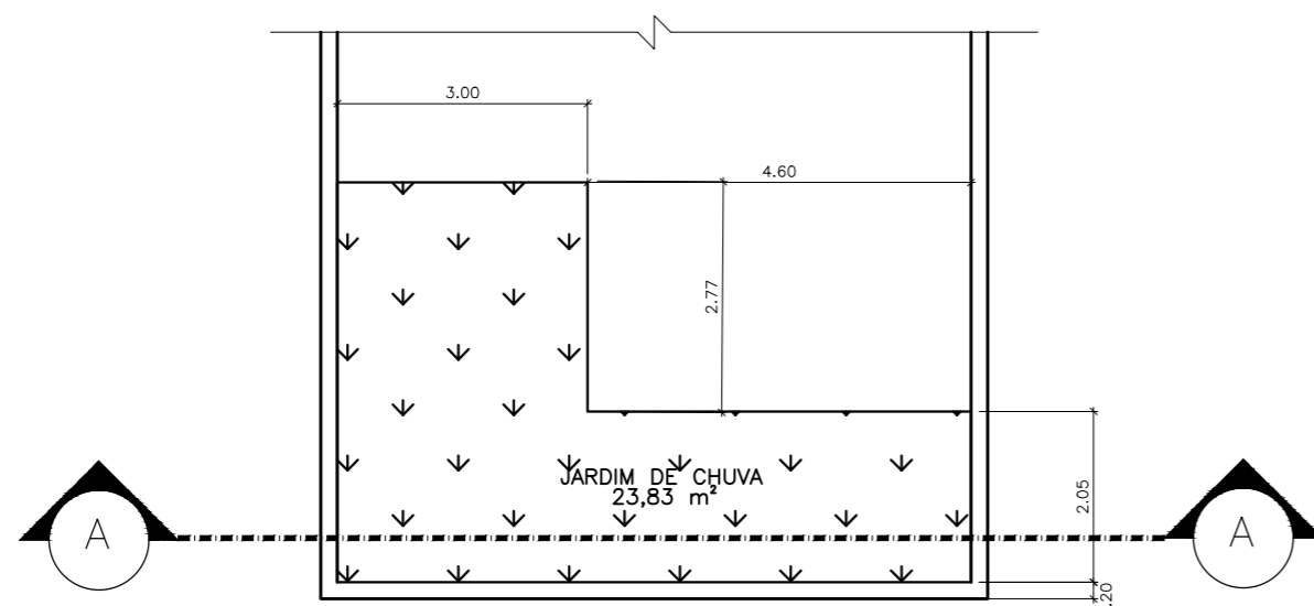
JARDIM DE CHUVA PLANTA BAIXA ESCALA 1:50
