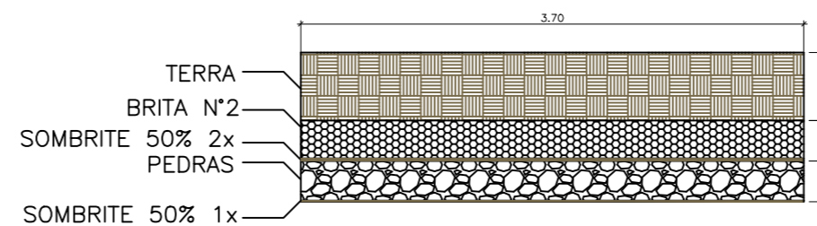
JARDIM DE CHUVA CORTE A-A ESCALA 1:20
