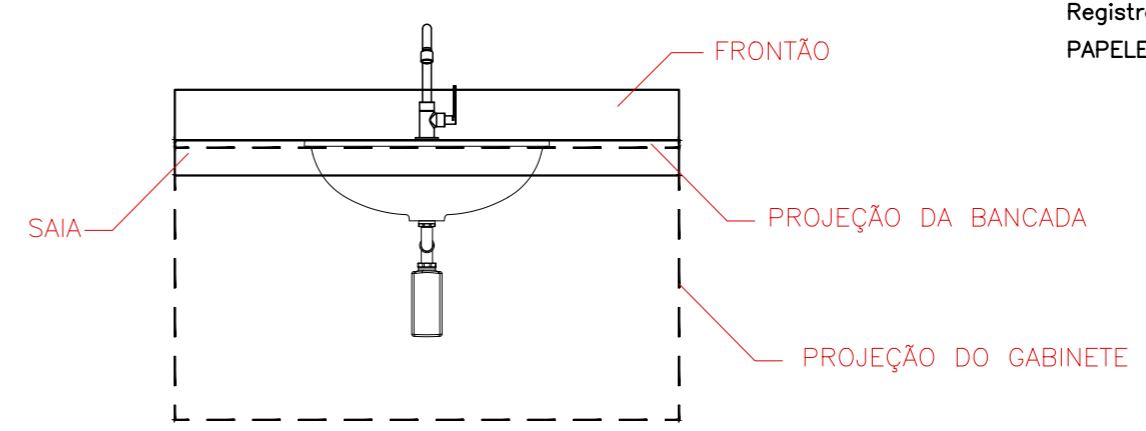
BANCADA W.C.1
