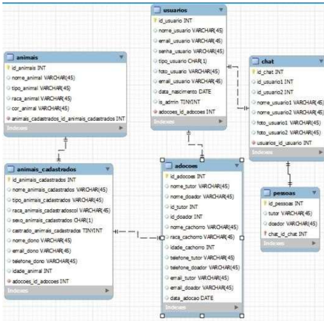
Figure 3: Diagrama de Entidade e Relacionamento
