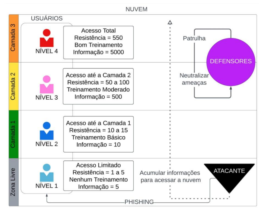
Figura 1 – Esquema dos agentes.
