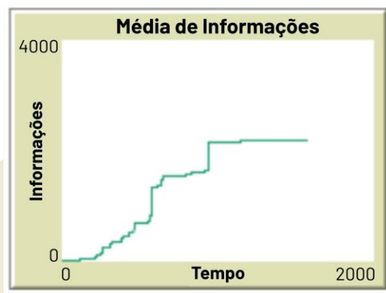
Figura 6 – Gráfico da quantidade média de informações acumuladas pelos atacantes em relação ao tempo.
