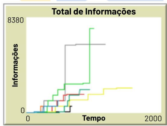
Figura 5 – Gráfico da quantidade total de informações acumuladas pelos atacantes em relação ao tempo.
