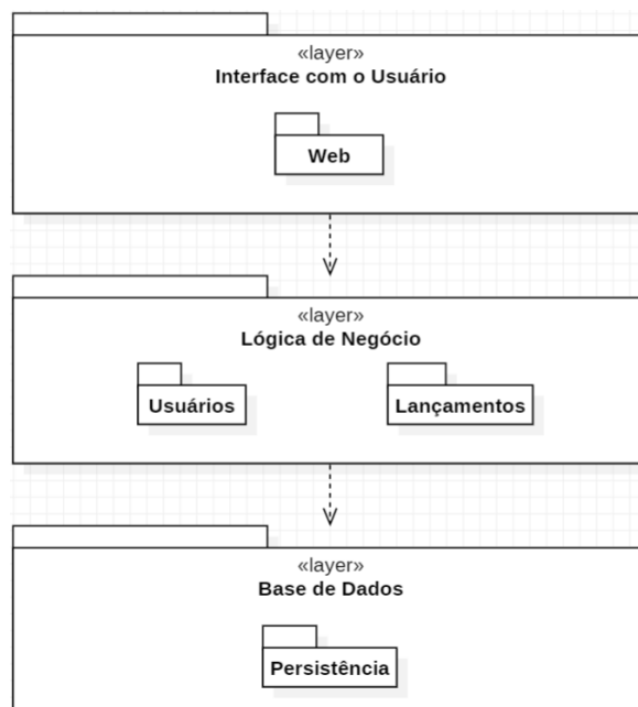
Figura 24 – Diagrama de pacotes da arquitetura lógica.
