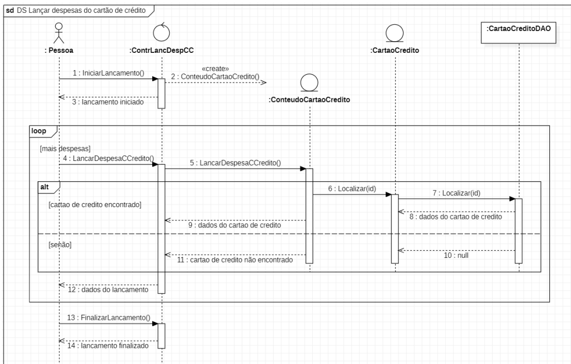
Figura 19 – Diagrama de interação Lançar despesas do cartão de crédito.
