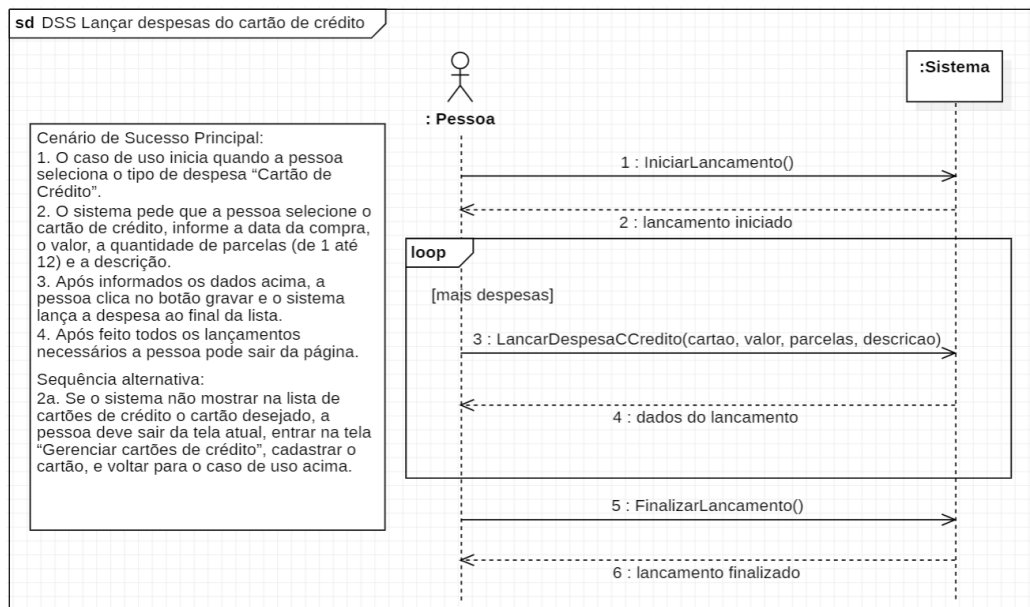
Figura 13 – Diagrama de Sequência de Eventos Lançar despesas do cartão de crédito.
