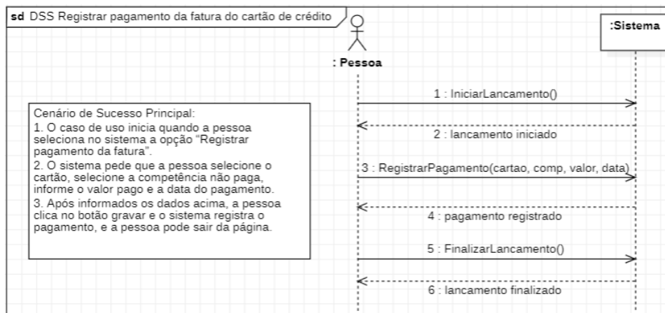
Figura 14 – Diagrama de Sequência de Eventos Lançar despesas do cartão de crédito.
