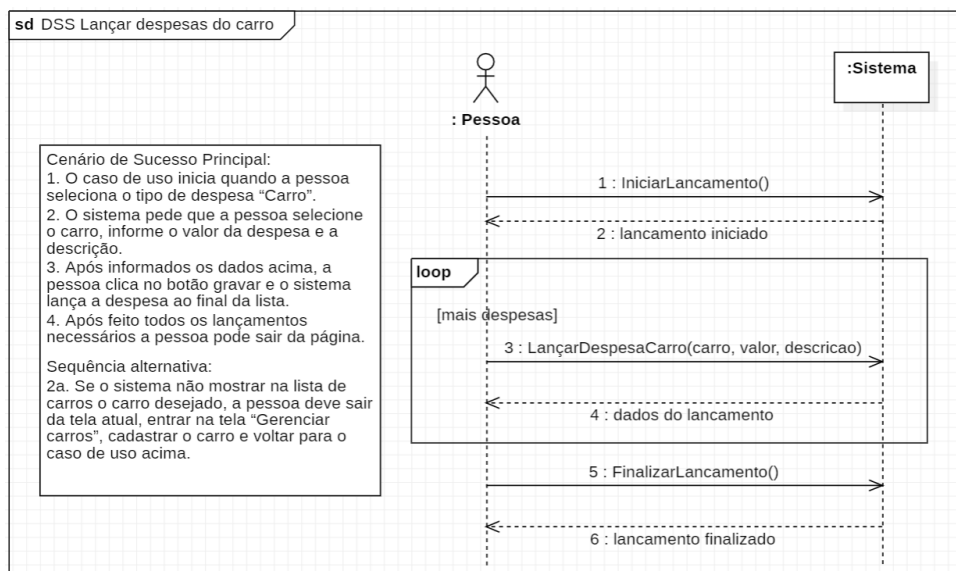
Figura 15 – Diagrama de Sequência de Eventos Lançar despesas do carro.
