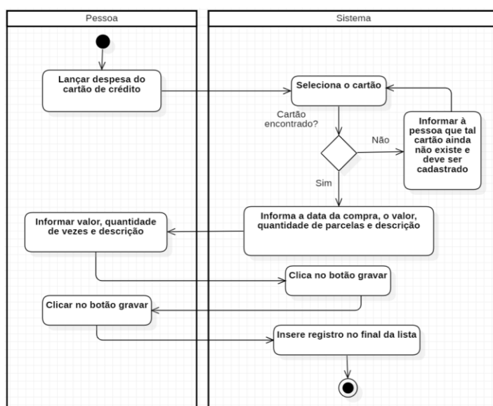
Figura 9 – Diagrama de atividade Lançar despesa do cartão de crédito.
