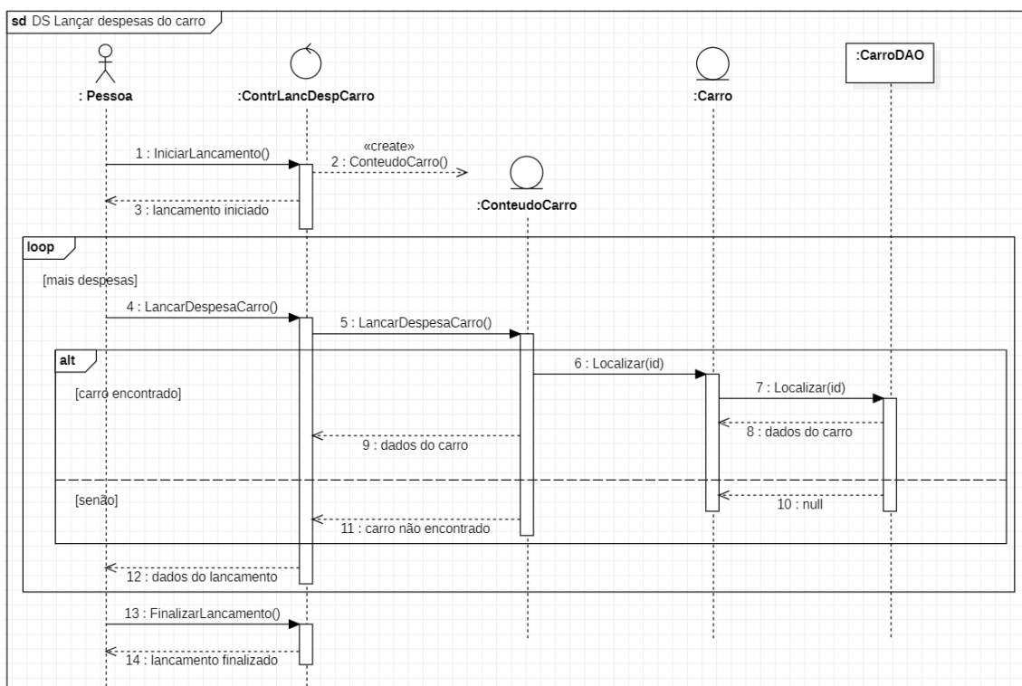
Figura 21 – Diagrama de interação Lançar despesas do carro.
