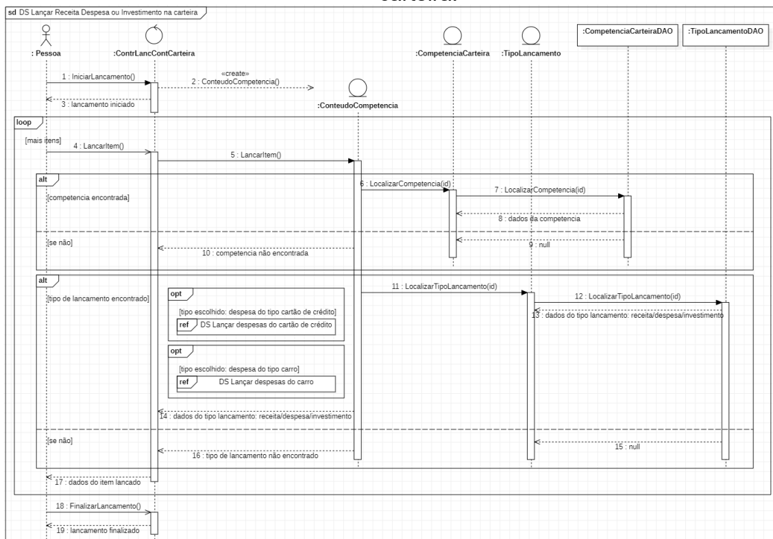
Figura 18 – Diagrama de interação Lançar receita, despesa ou investimento na carteira.
