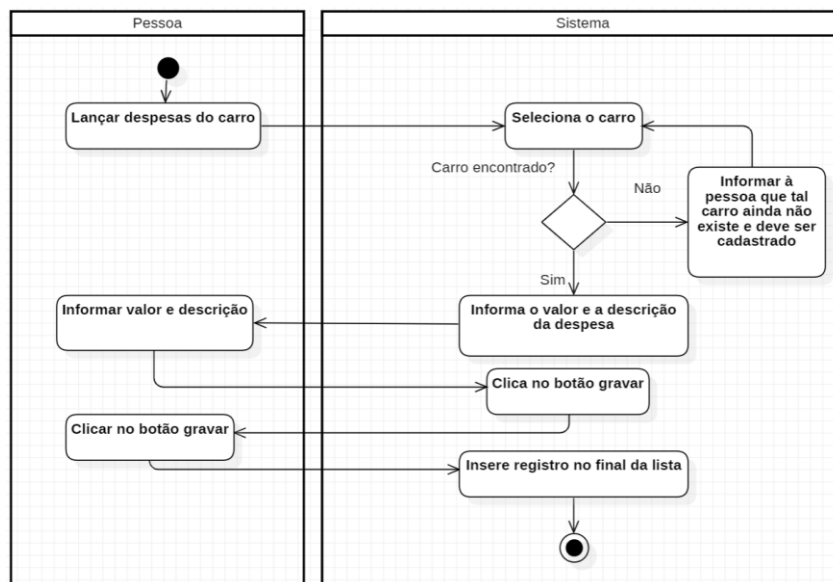
Figura 10 – Diagrama de atividade Lançar despesa do carro.
