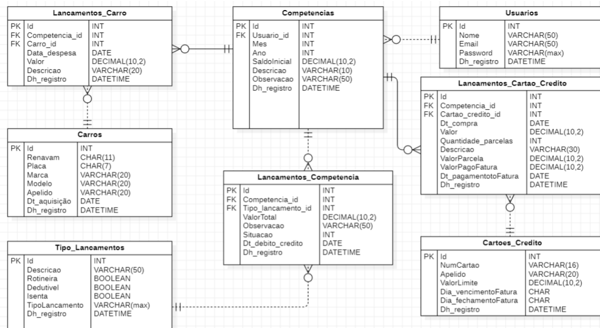
Figura 23 – Modelagem da base de dados.
