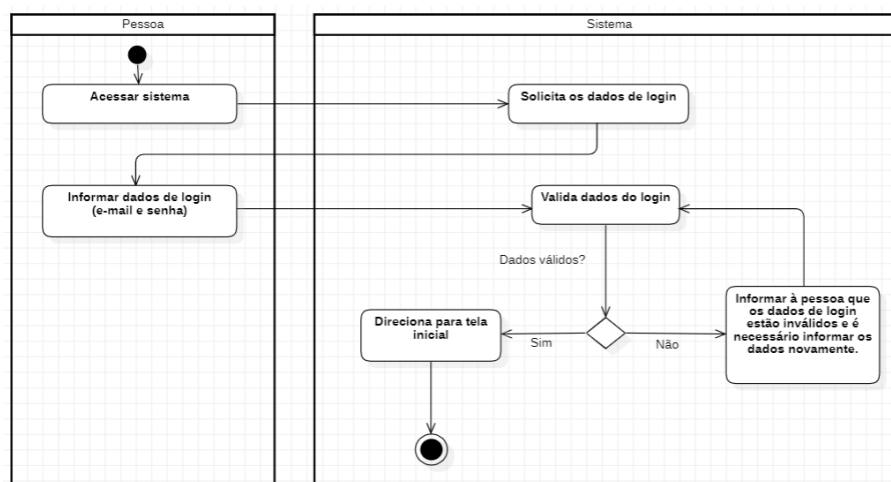
Figura 7 – Diagrama de atividade Logar no sistema.
