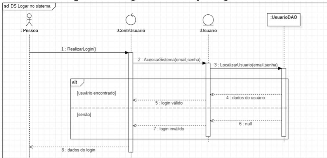
Figura 17 – Diagrama de interação Logar no sistema.
