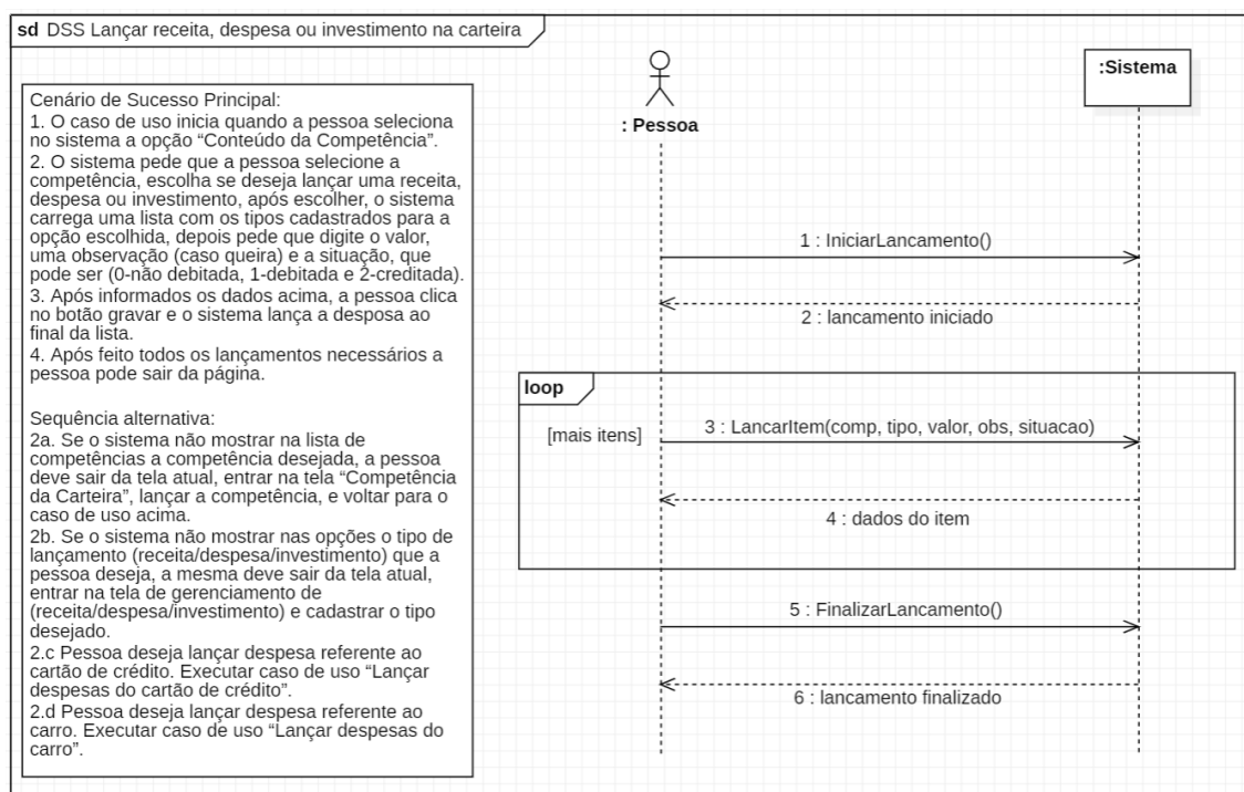
Figura 12 – Diagrama de Sequência de Eventos Lançar receita, despesa ou investimento na carteira.
