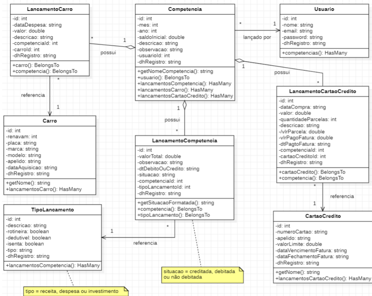
Figura 22 – Diagrama de classes.
