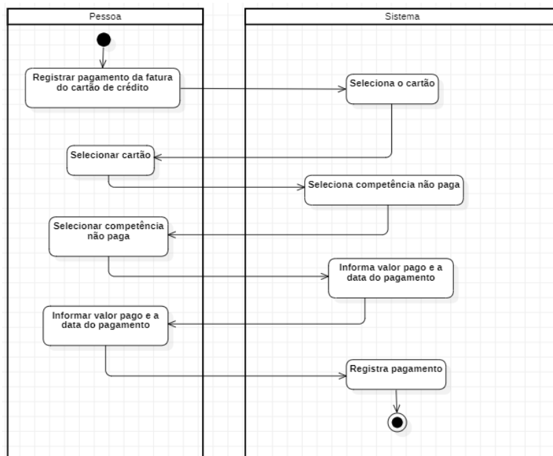
Figura 10 – Diagrama de atividade registrar pagamento da fatura do cartão de crédito.
