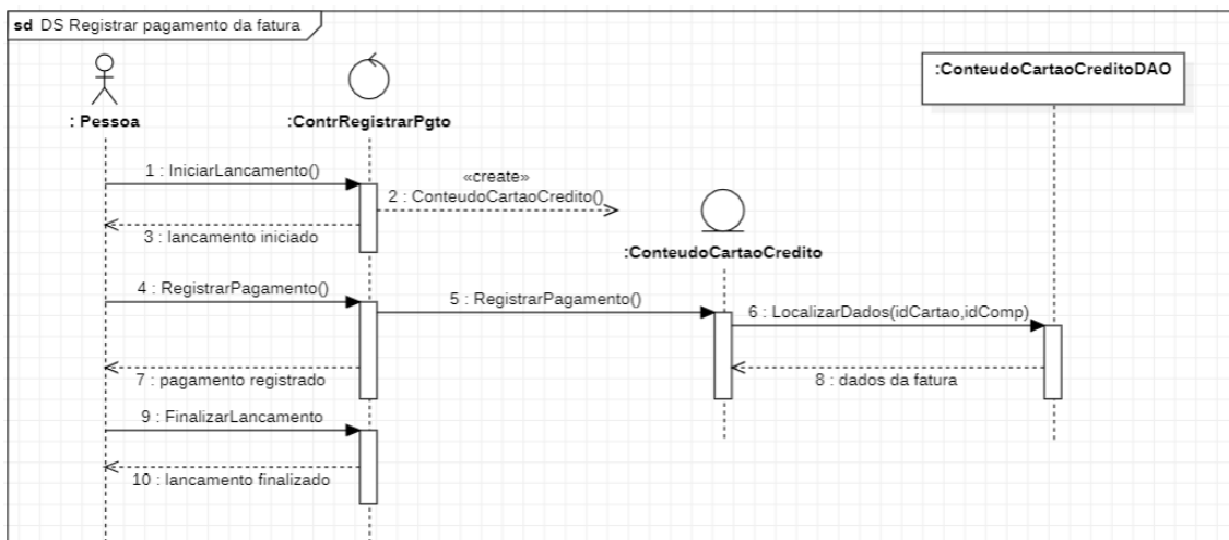
Figura 20 – Diagrama de interação Registrar pagamento da fatura.
