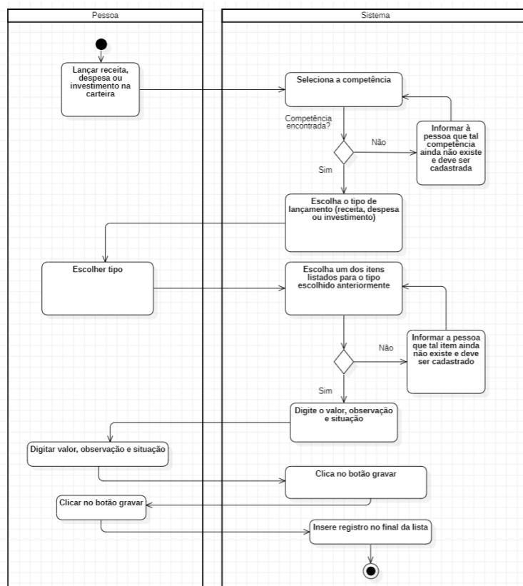
Figura 8 – Diagrama de atividade Lançar receita, despesa ou investimento na carteira.
