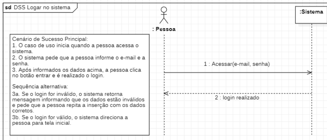
Figura 11 – Diagrama de Sequência de Eventos Logar no sistema.
