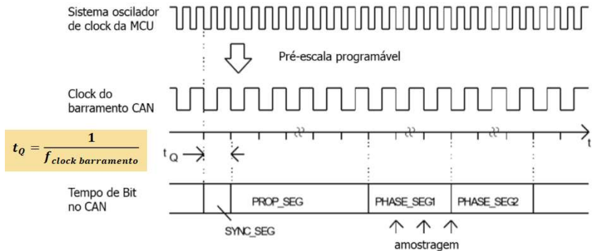
Figura 19 – Pré-escala programável
