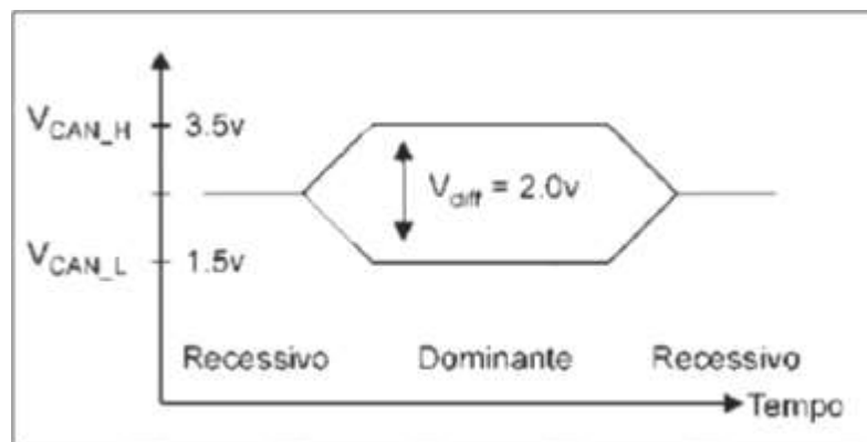
Figura 3 – Bits dominantes e recessivos no barramento CAN
