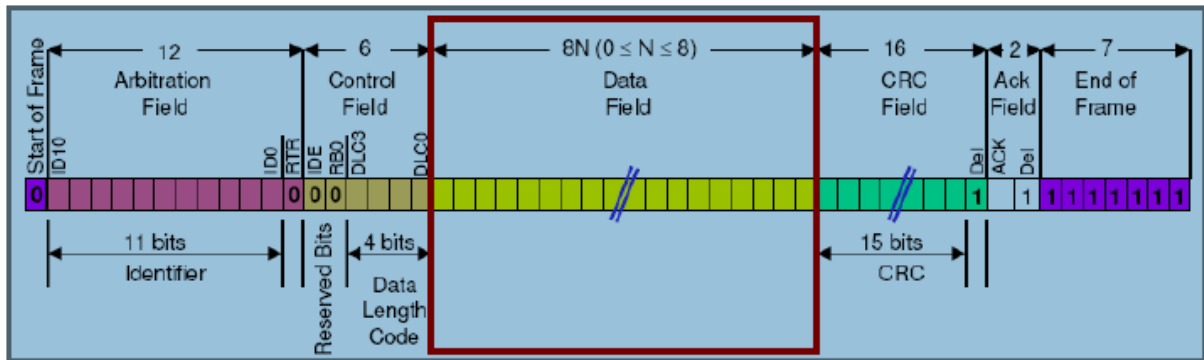
Figura 13 -- Campo de Dados em Evidência
