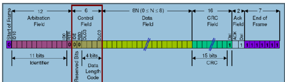
Figura 12 -- Campo de Controle em Evidência
