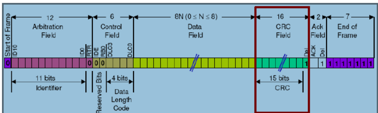
Figura 14 -- Campo de CRC em Evidência
