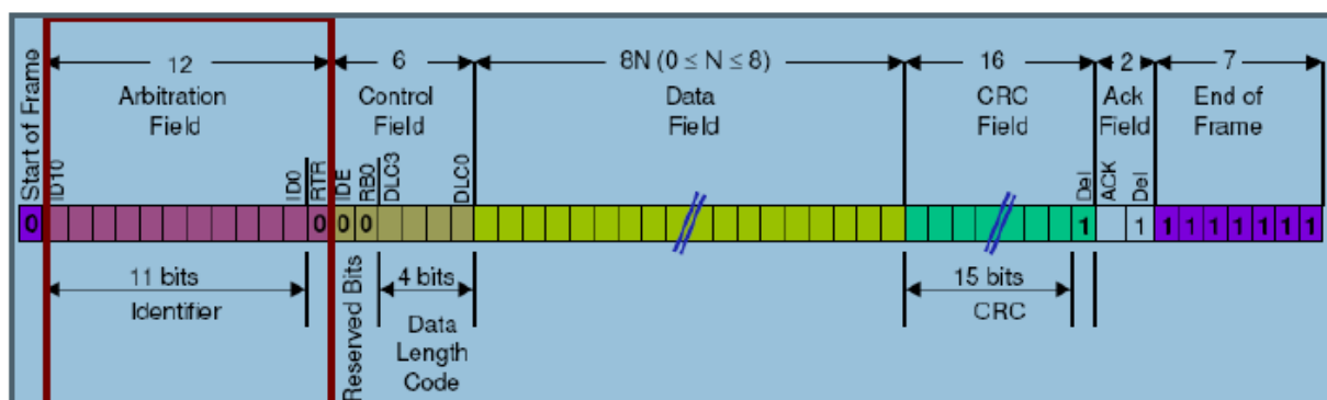
Figura 10 -- Campos de Arbitragem, Identificador 11 bits e RTR em Evidência
