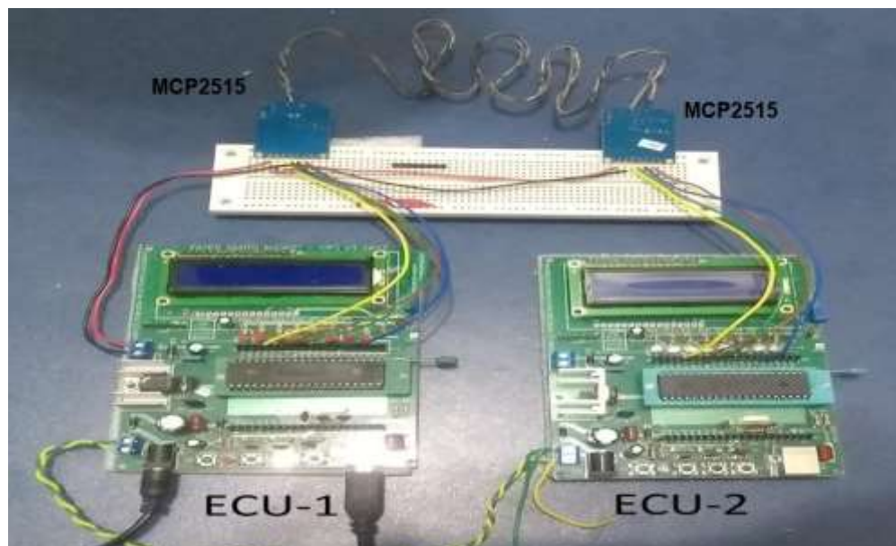
Figura 22– Setup do projeto
