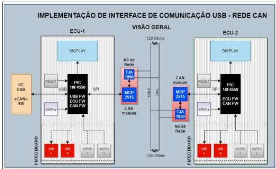
Figura 1 – Diagrama da arquitetura da rede CAN proposta
