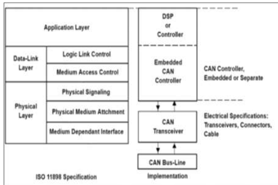
Figura 6 -- Protocolos da Camada Física
