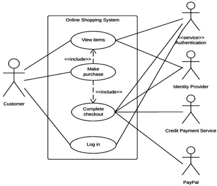
Figura 5- DIAGRAMA USE CASE
