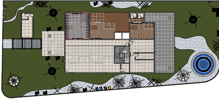
1 terreo 1:100
