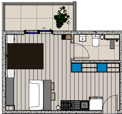
5 Ap. Tipo 1:25
