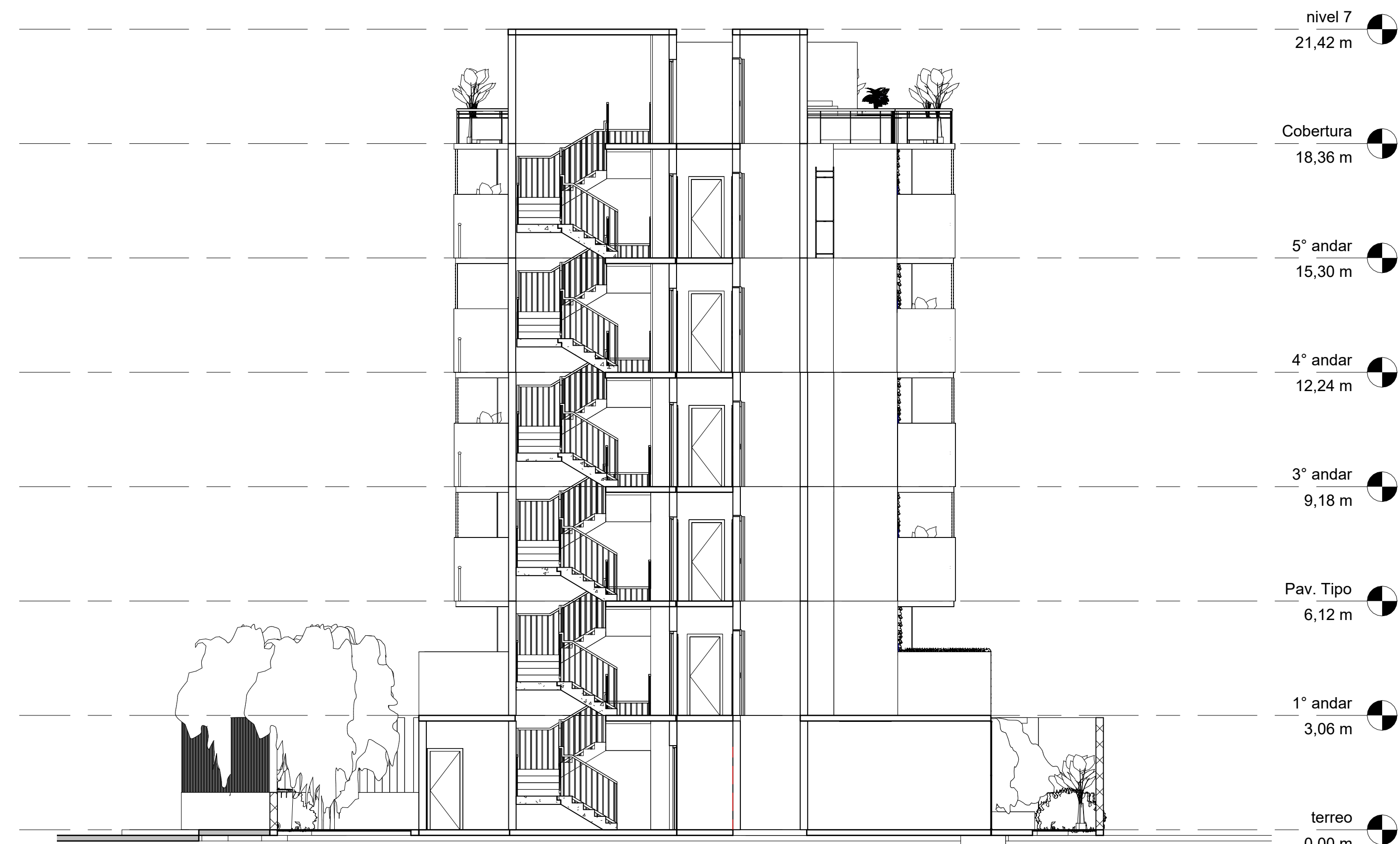
3 CC 1 : 100
