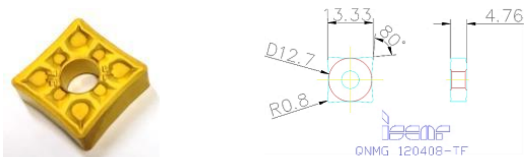
Figura 25 - Inserto QNMG 120408 - TF
