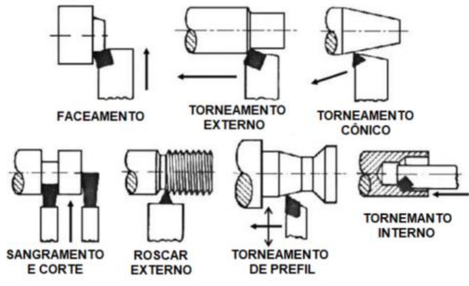
Figura 5 - Operações mais comuns de torneamento.
