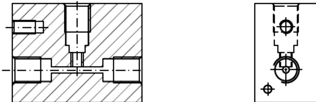
Figura 19 - Projeto em CAD do bloco misturador da névoa
