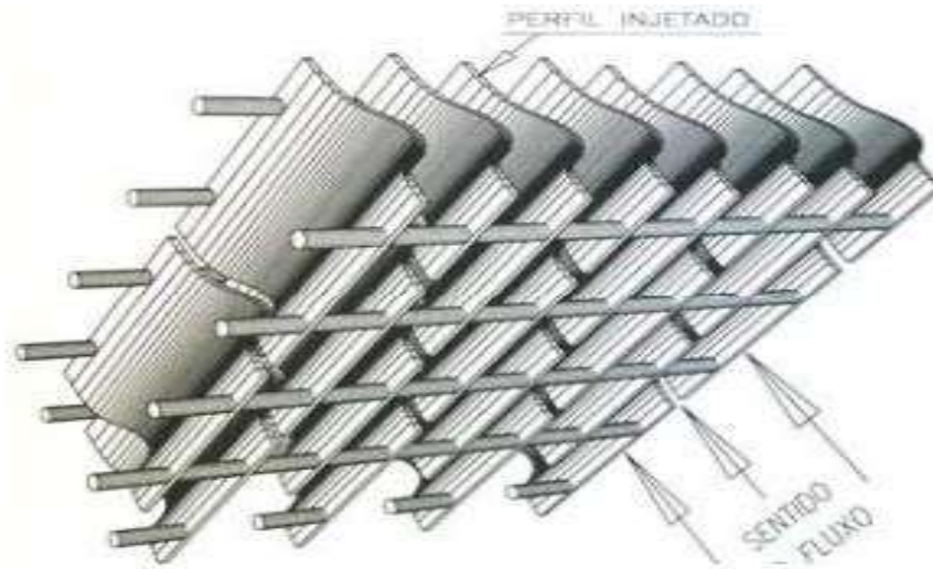
Figura 3.10 - Eliminador de Gotas
