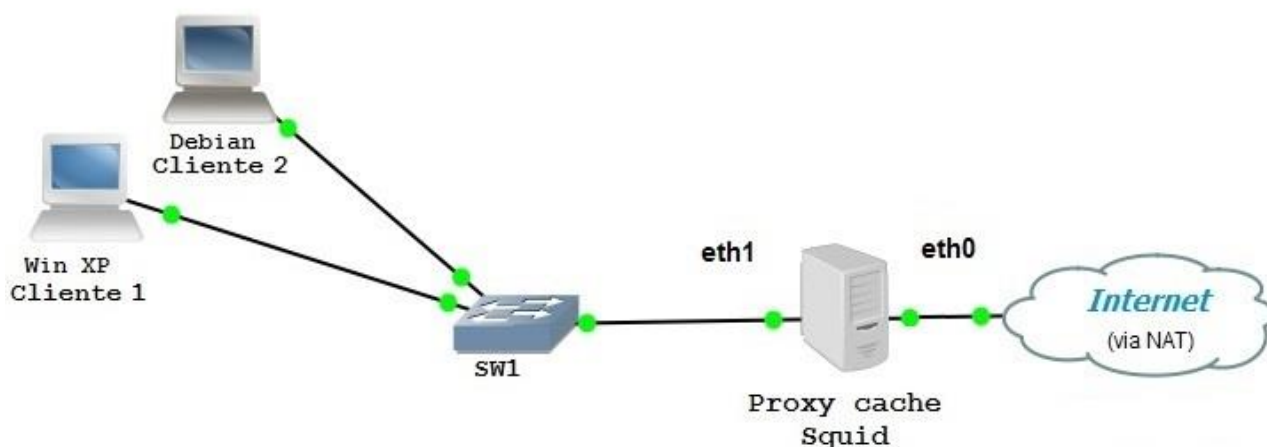
Figura 2: Ilustração do ambiente de testes utilizando Squid
