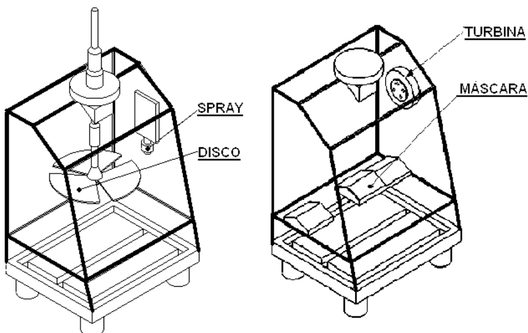
Figura 15: Pulverização de corante
