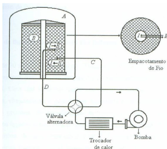
Figura 4: Esquema representativo de tingimento de bobinas
