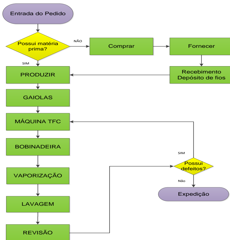
Figura 12: Fluxograma de Produção
