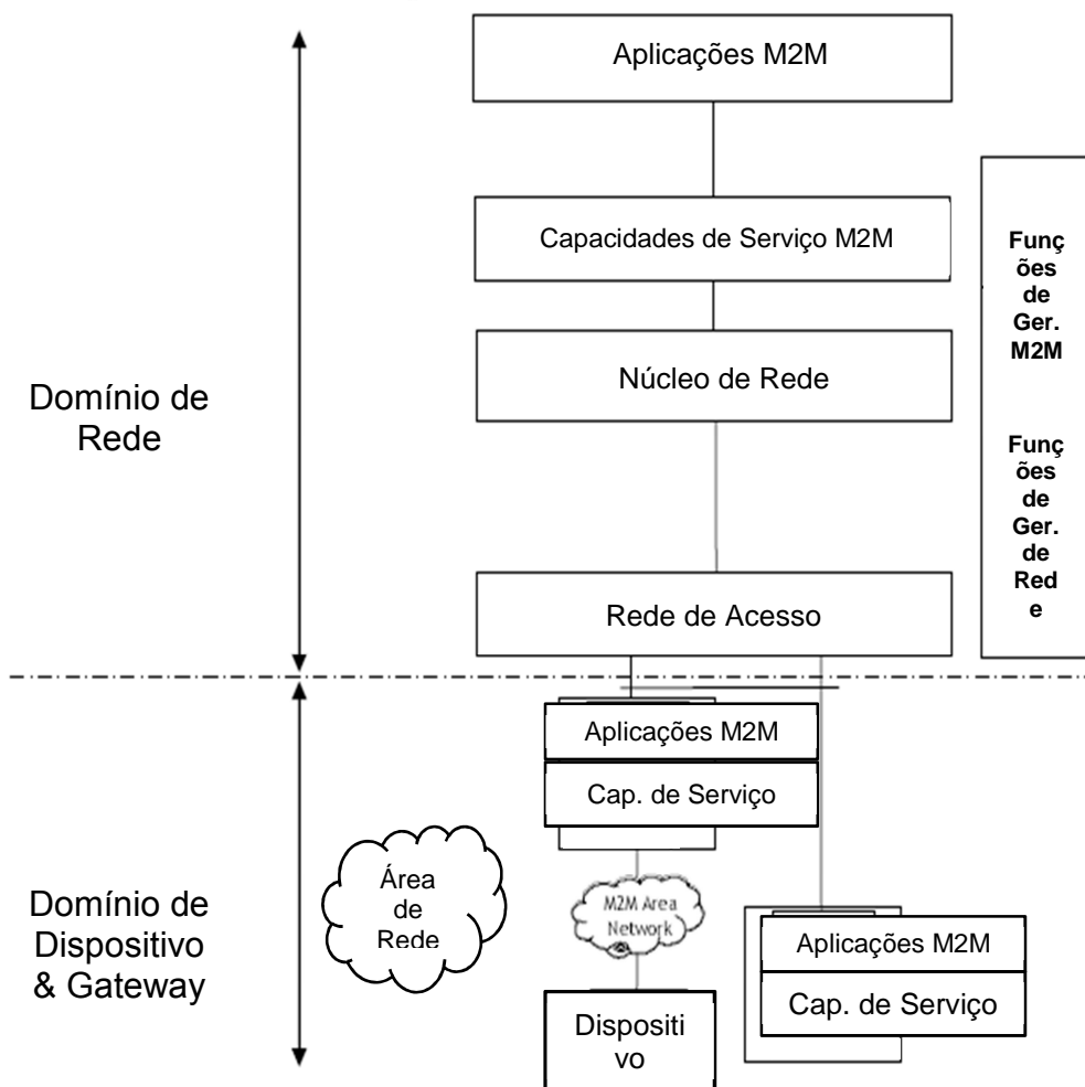
Figura 4: Arquitetura M2M
