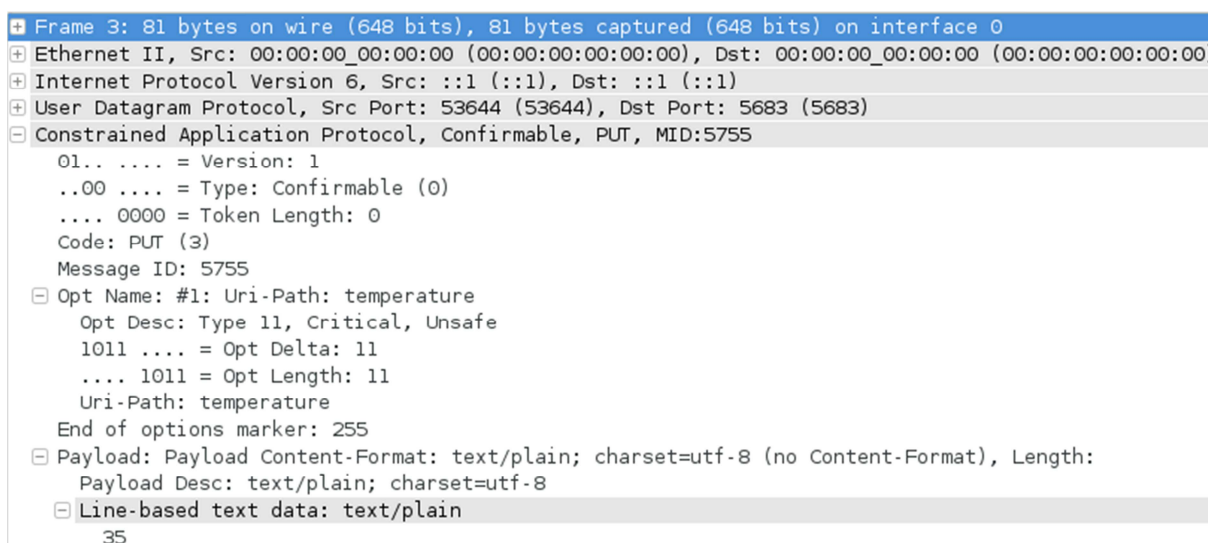
Figura 24: Payload do pacote da requisição PUT
