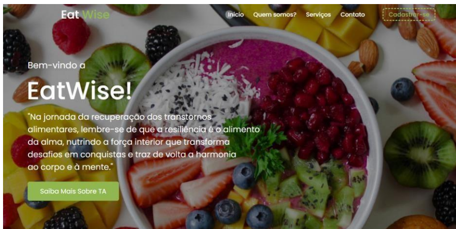
FIGURA 1 - PÁGINA
