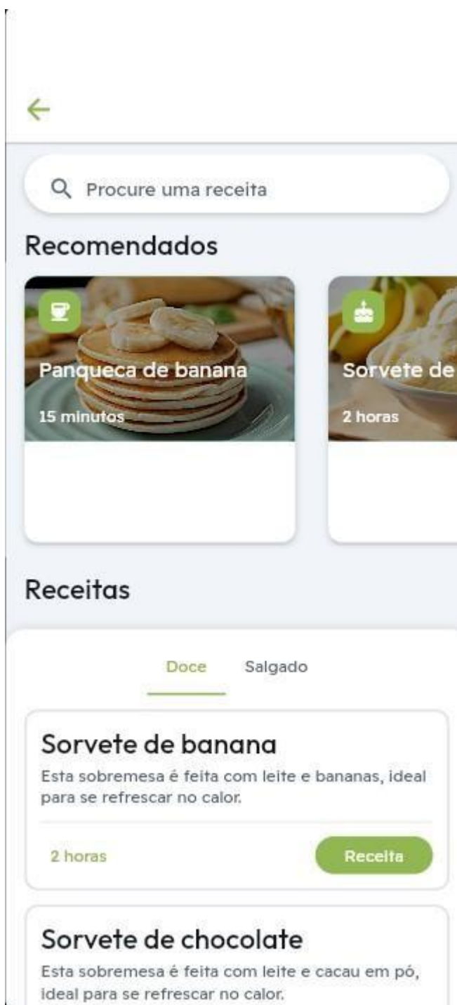
FIGURA 24– RECEITA (MOBILE)
