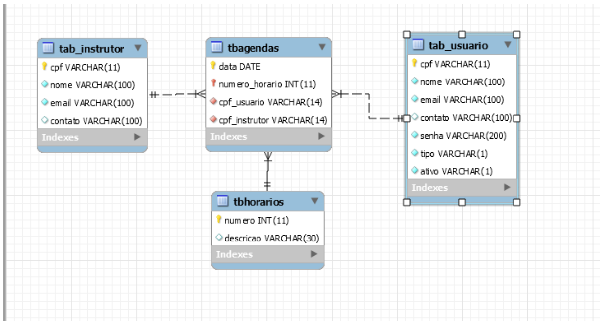
Figura 23: Relacionamento de tabela banco de dados
