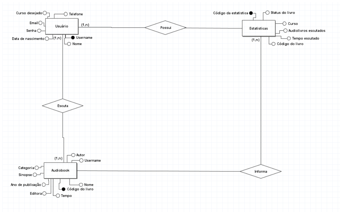
Figura 26: MER do projeto LIA.
